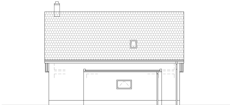
POHLED BOČNÍ
